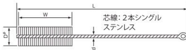
HN-120シリーズ 極細管 φ1.5～φ4.0 全長120mm
